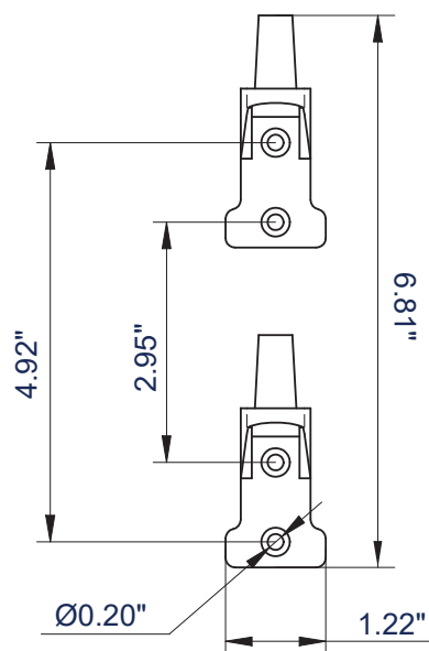
WALL HINGES
