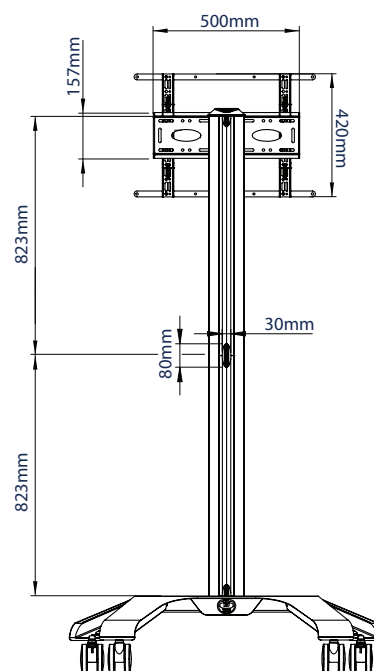
RÜCKANSICHT
